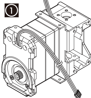
接続ケーブル (ZH接続ケーブル 2 A 200mm)
