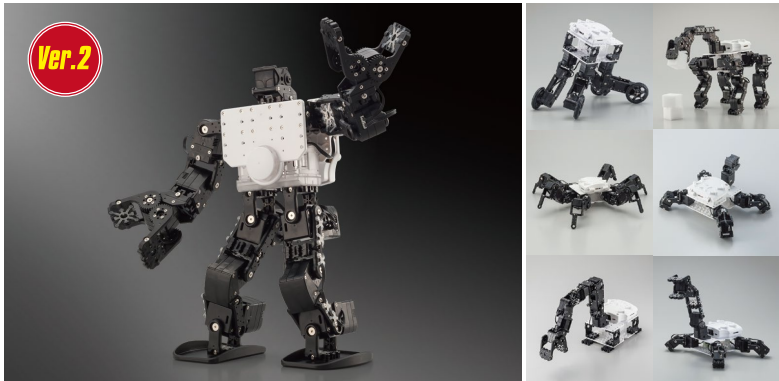
KXR アドバンスセットA Ver.2 価格:オープン No.03158 フルセットのアドバンスセットAがVer.2に進化。サーボのトルクアップでさらに安定性が増しました。セットのパーツが増量し組換えの自由度も増えました。ハイトルクサーボが6コ個付属します。
